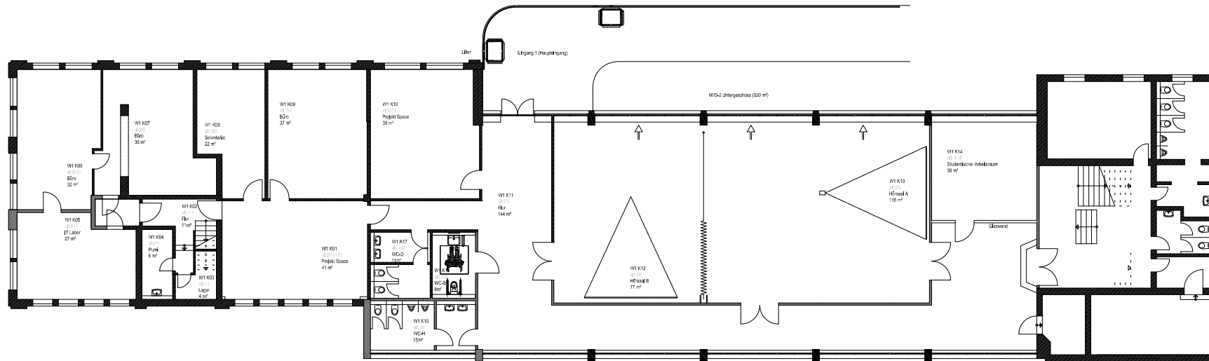
Gebäude W1 Grundriss UG M1:100
