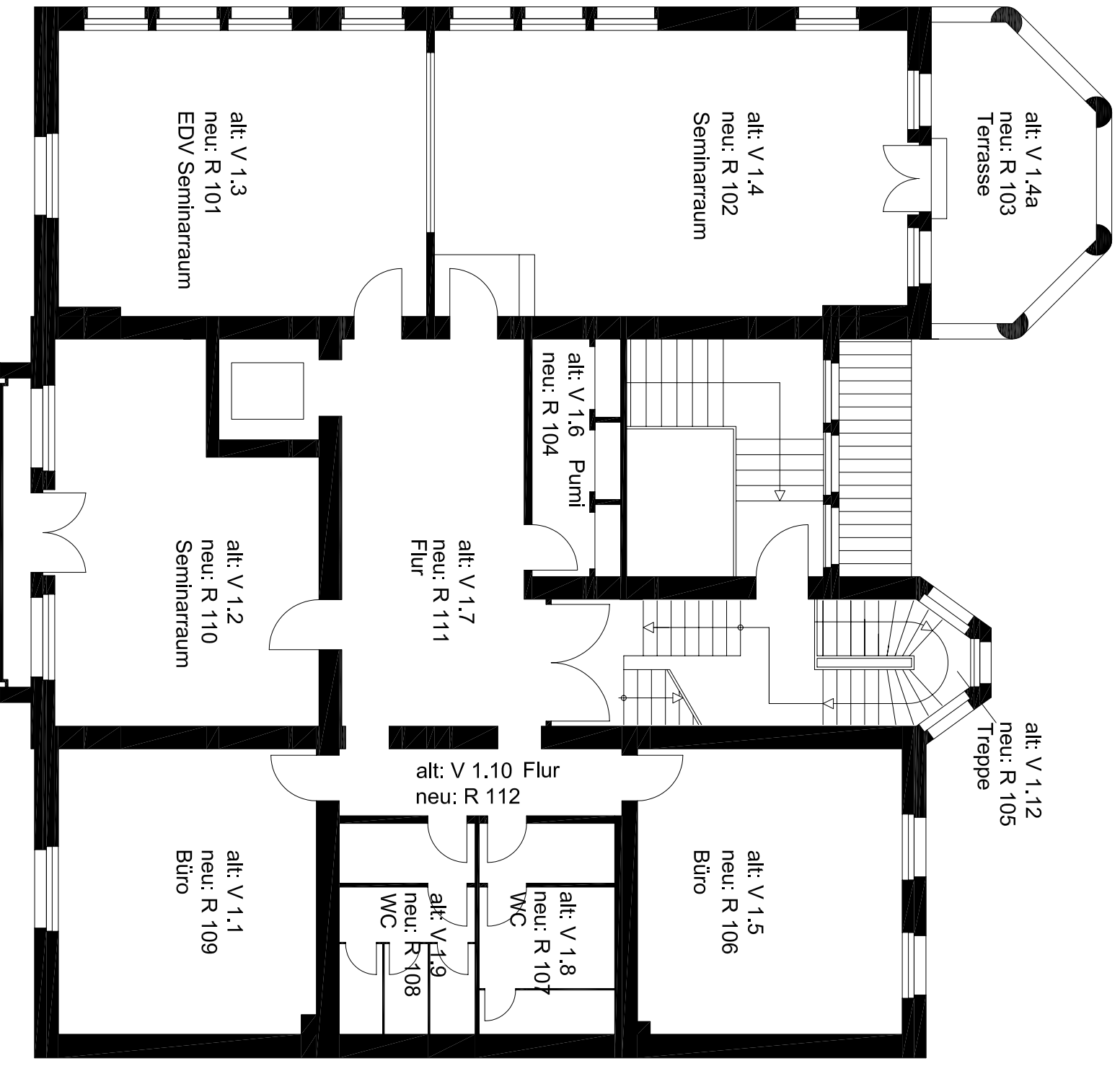
Gebäude R 1. Obergeschoss
