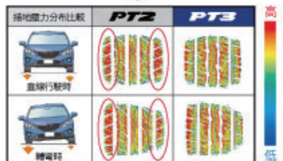
PT2壓力集中在胎面 PT3壓力分布更加均勻，接地感提高
