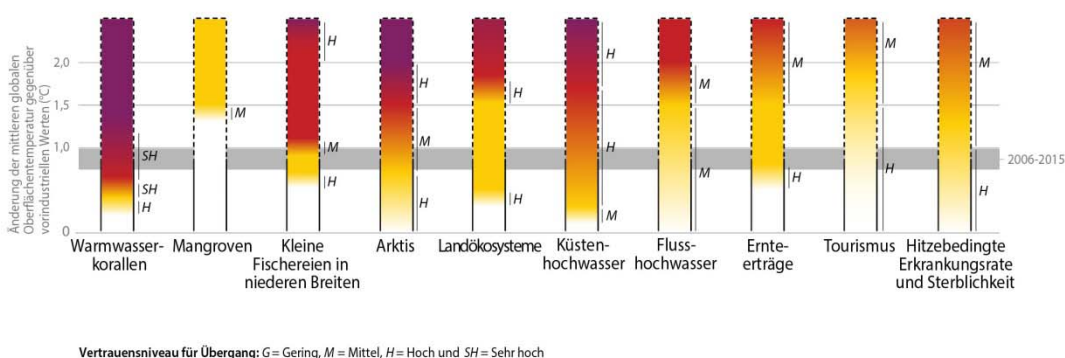
Abbildung SPM.2: Fünf Gründe zur Besorgnis ( Reasons for Concern, RFCs ) liefern einen Rahmen für die Zusammenfassung von Schlüsselfolgen und -risiken über Sektoren und Regionen hinweg; sie wurden im Dritten IPCC-Sachstandsbericht eingeführt. RFC veranschaulichen die Auswirkungen der globalen Erwärmung für Menschen, Wirtschafts- und Ökosysteme. Folgen und/oder Risiken für jeden RFC beruhen auf der Bewertung der neu erschienenen Literatur. Wie im AR5 wurde diese Literatur genutzt, um zu Expertenbeurteilungen über die Niveaus globaler Erwärmung zu kommen, bei denen das Ausmaß an Folgen und/oder Risiken jeweils nicht nachweisbar, moderat, hoch oder sehr hoch sind. Die Auswahl von Folgen und Risiken für natürliche, bewirtschaftete und menschliche Systeme im unteren Teil der Abbildung ist beispielhaft und erhebt keinen Anspruch auf Vollständigkeit. {3.4, 3.5, 3.5.2.1, 3.5.2.2, 3.5.2.3, 3.5.2.4, 3.5.2.5, 5.4.1, 5.5.3, 5.6.1, Box 3.4}
