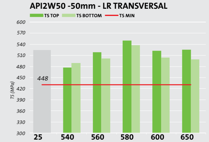
Gráfico 8 - Variação do limite de resistência (MPa) com o aumento de temperatura (°C) após tratamento térmico SPWHT. Fonte: Usiminas
