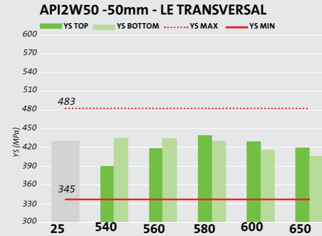
Gráfico 7 - Comportamento do aço API 2W-50 após ensaio PWHT
