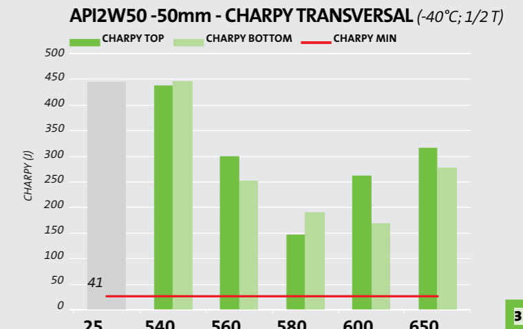
Gráfico 10 - Variação da energia de absorção ao impacto (J) com o aumento de temperatura (°C) após tratamento térmico SPWHT. Fonte: Usiminas
