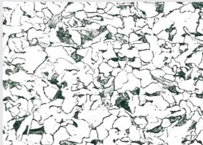
Figura 3 – Microestrutura de aço 50 kJ/mm 2 ; espessura: 25 mm do processo convencional versus CLC (x200). Fonte: Usiminas
