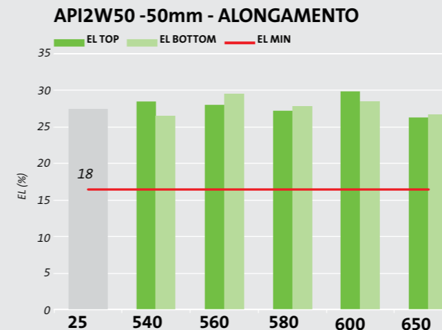
Gráfico 9 - Variação do Alongamento (%) com o aumento de temperatura (°C) após tratamento térmico SPWHT. Fonte: Usiminas
