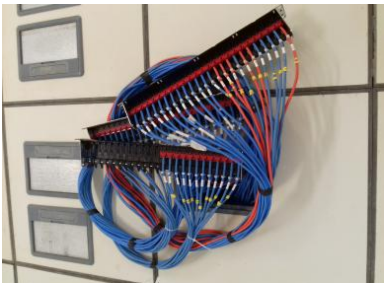
Cabos UTP CAT6 conectados aos patch panel e certificados
