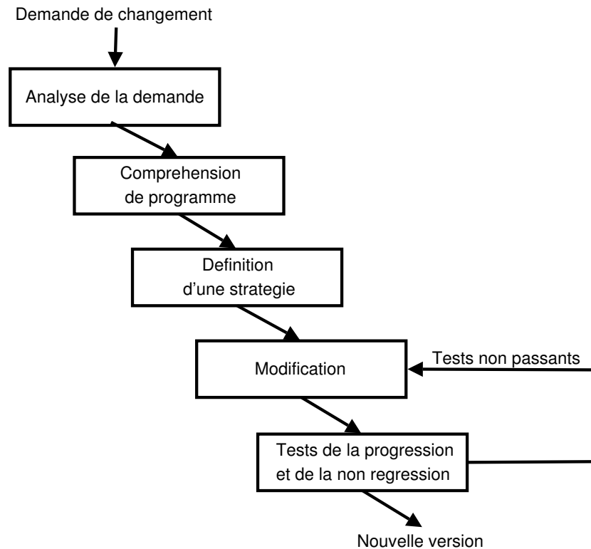
FIG. 2.3 – Micro-processus d'évolution
