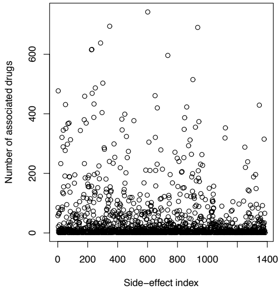
Index-plot
