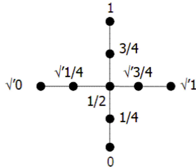
Fig. 2.2. \text{Rt}(\mathbf{L}_5) .
