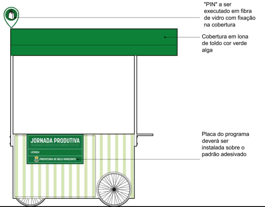
CARRO FRUTAS - VISTA LATERAL
