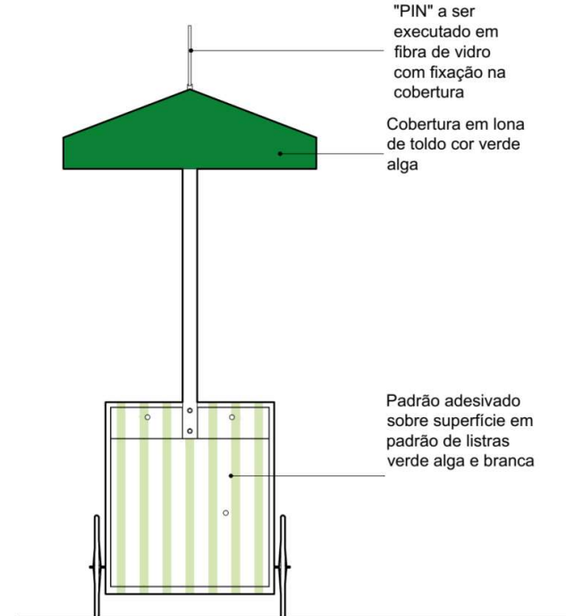
CARRO FRUTAS - VISTA FRONTAL
