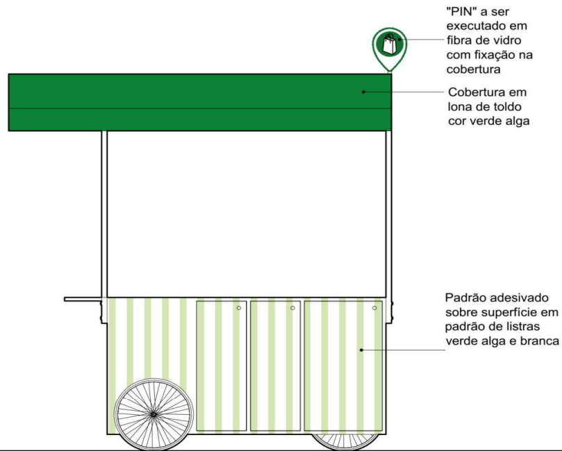
CARRO FRUTAS - VISTA LATERAL ESCALA 1/25
