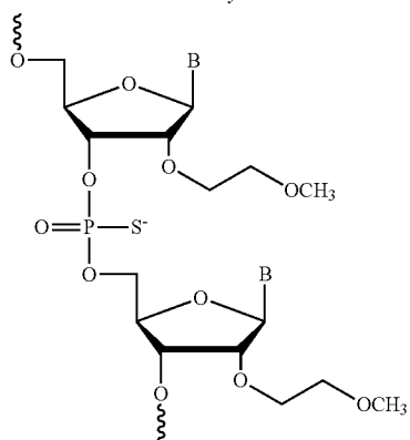
2'O-MOE PS
