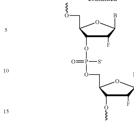
2'-F PS
