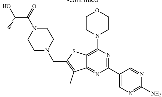
apitolisib
