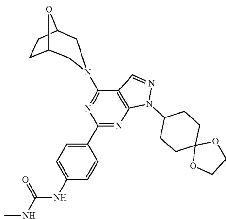
WYE-125132
