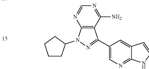
PP 121
