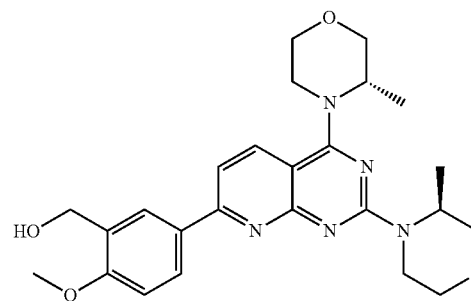
AZD 8055
