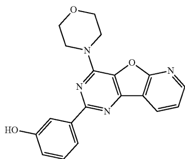
PI-103
