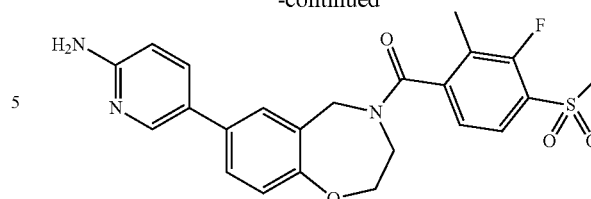
XL 388
