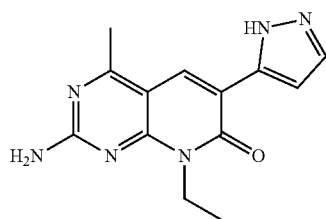
XL765 (voxtalisib)
