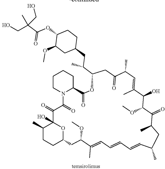
temsirolimus
