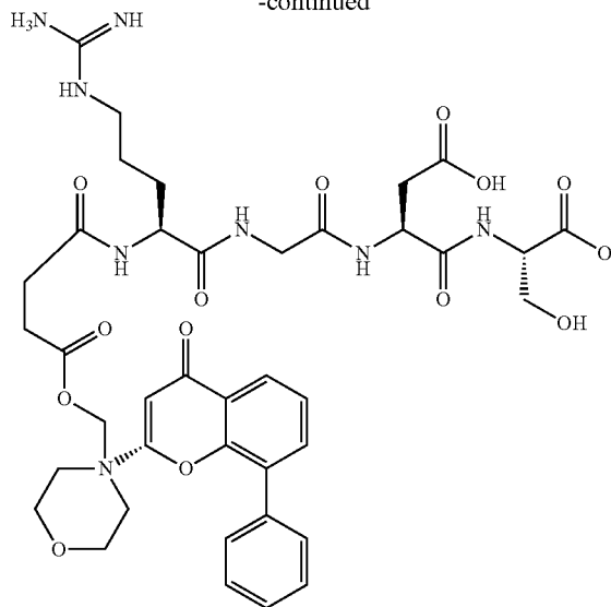
SF1126
