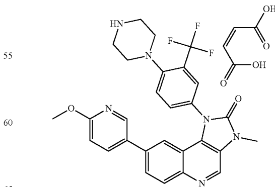
BGT226
