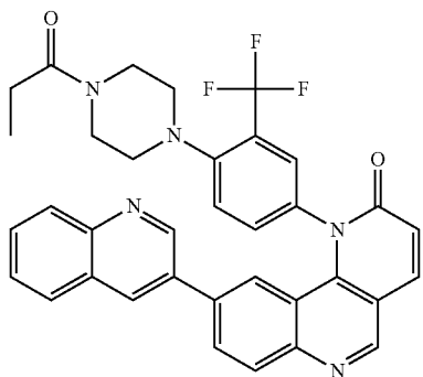
torin-1
