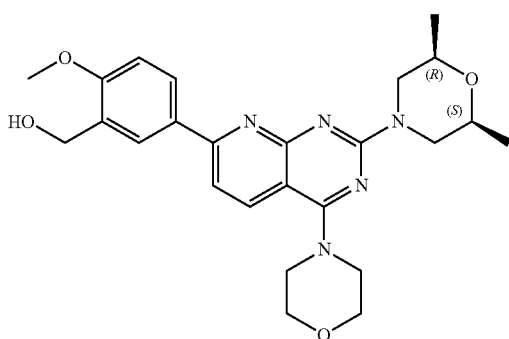
KU-0063794
