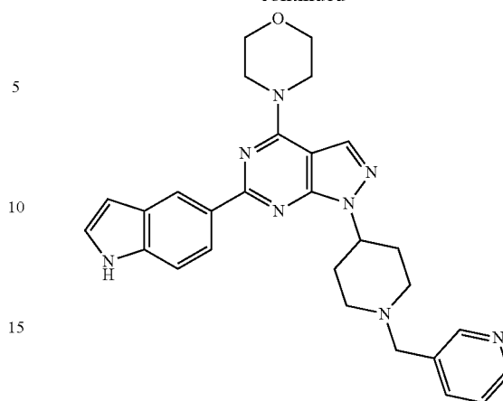
WAY 600
