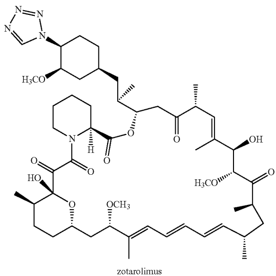
zotarolimus
