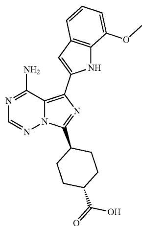
OSI 027
