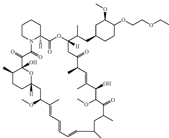
umirolimus
