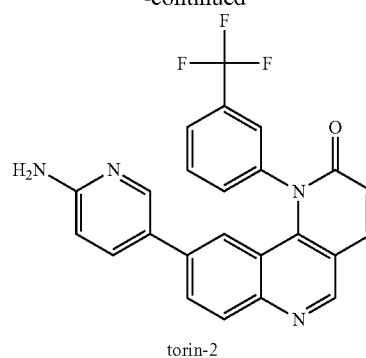
torin-2
