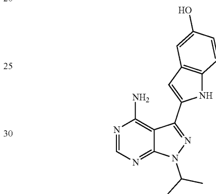
torkinib
