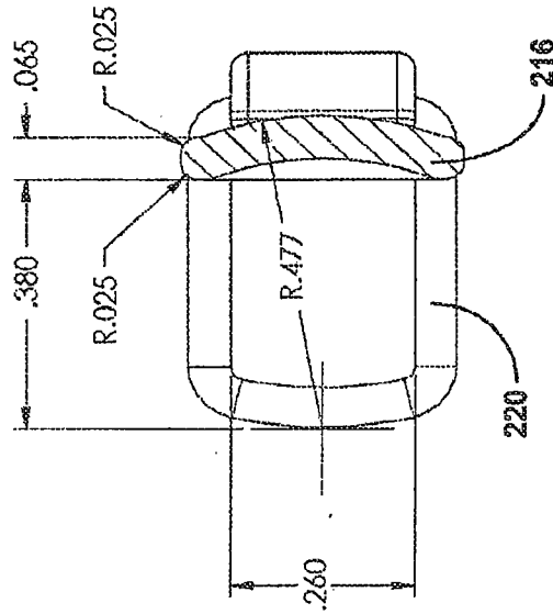
SECTION D-D
