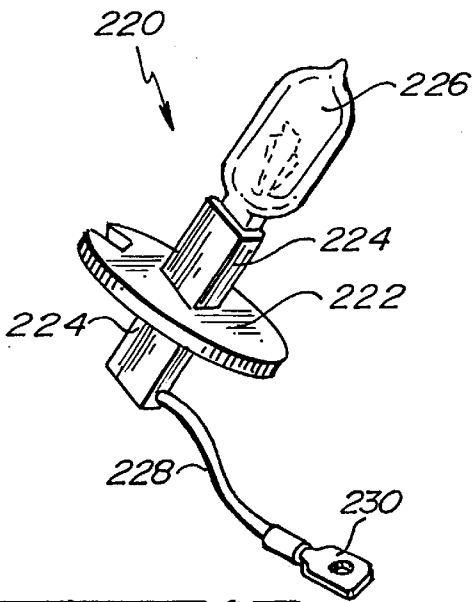
Fig. 18. PRIOR ART
