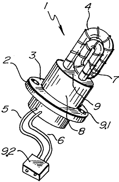
Fig. 16. PRIOR ART
