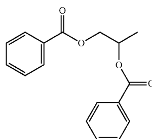
Propylene Glycol Di-Benzoate
