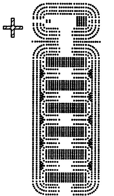
CONTACTS FIG. 16A-6
