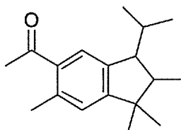
Traseolide (Quest)
