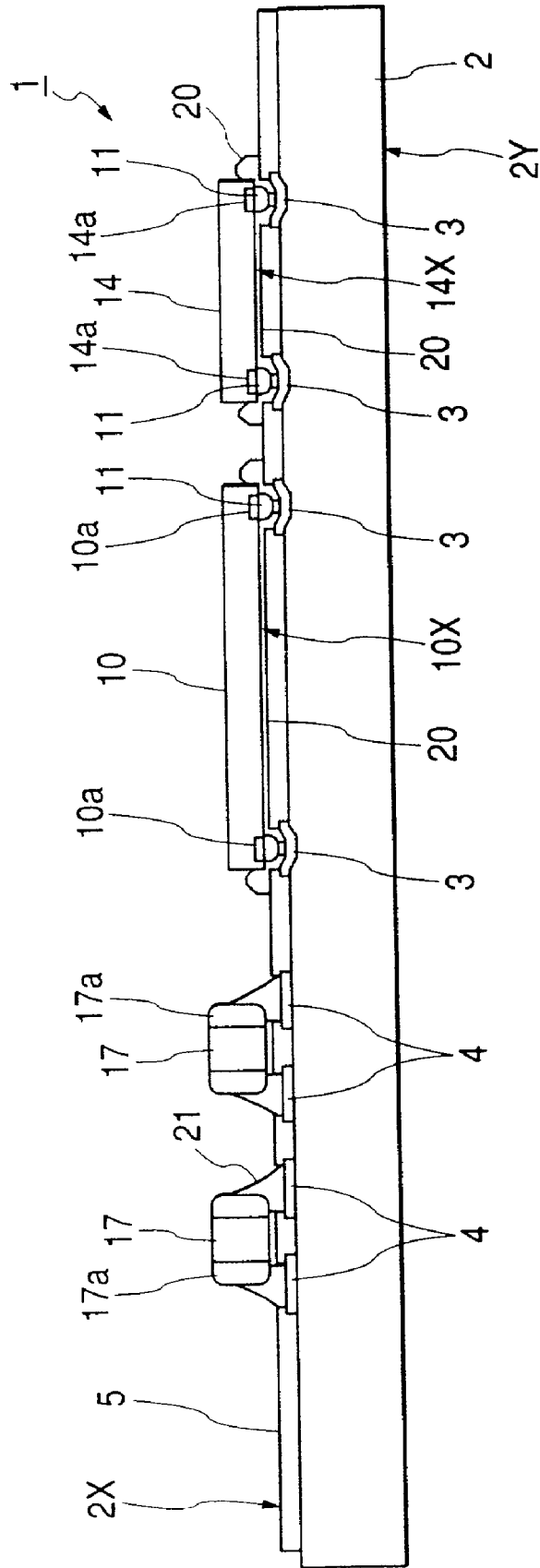
FIG. 15
