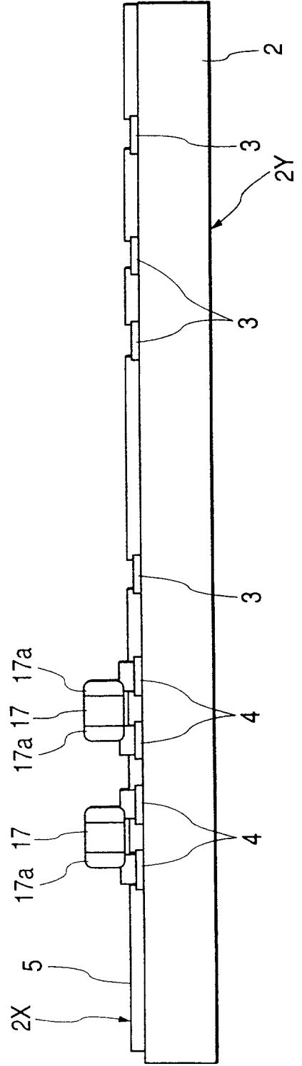
FIG. 11(B)
