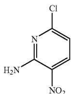
6-Chloro-3-nitropyridin-2-amine
