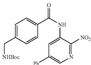
tert-Butyl(4-[[3-nitro-6-phenylpyridin-2-yl]amino]carbonyl)benzyl)carbamate
