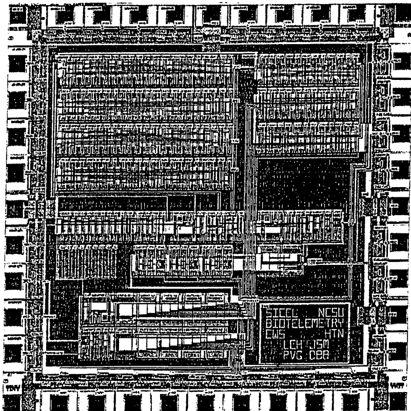
IC LAYOUT
