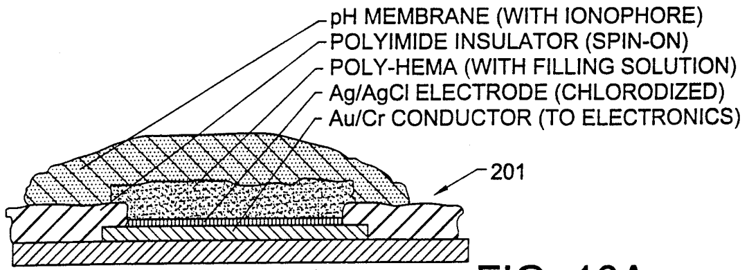
KAPTON® SUBSTRATE pH SENSOR ON KAPTON®
