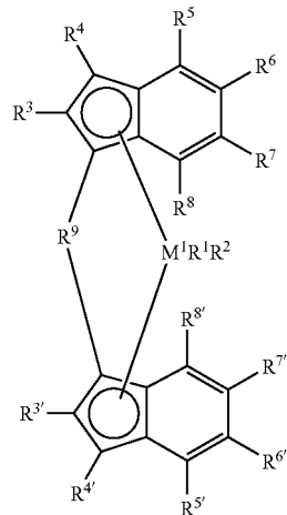
meso/pseudomeso isomer
