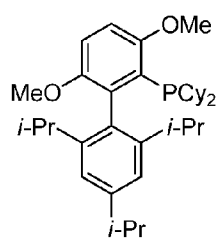
1, BrettPhos
