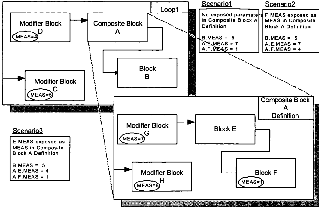
Figure 86 - Modifier Block Parameter override precedence
