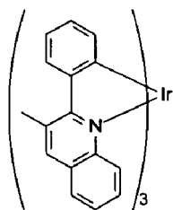
Ir(3-Mepq) 3
