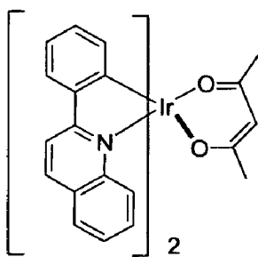
Ir(pq) 2 (acac)
