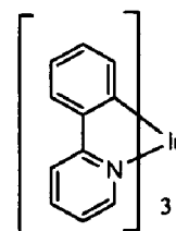
Ir(ppy) 3
