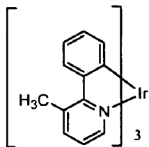
Ir(3-Meppy) 3
