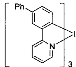
Ir(5-Phppy) 3
