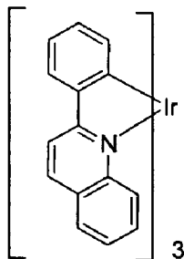
Ir(pq) 3
