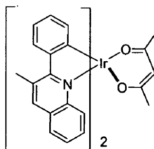
Ir(3-Mepq) 2 (acac)
