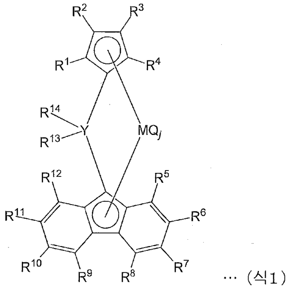
[화학식 3]
