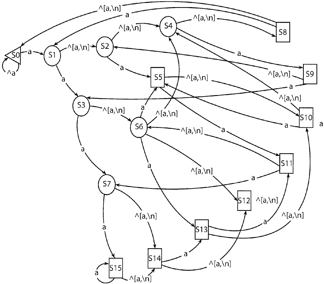
DFA for the pattern: ".*a[^\n][^\n][^\n]" Graph size of 16 nodes
