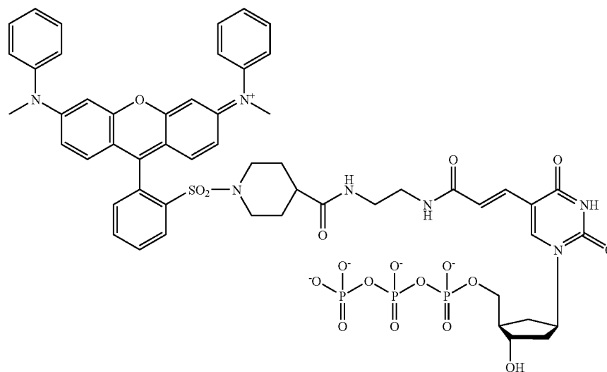
QSY 7 dTTP
