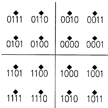
FIG. 12c 4 BITS PER BAUD
