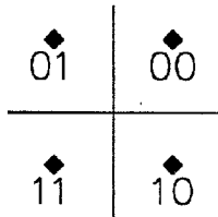
FIG. 12a 2 BITS PER BAUD
