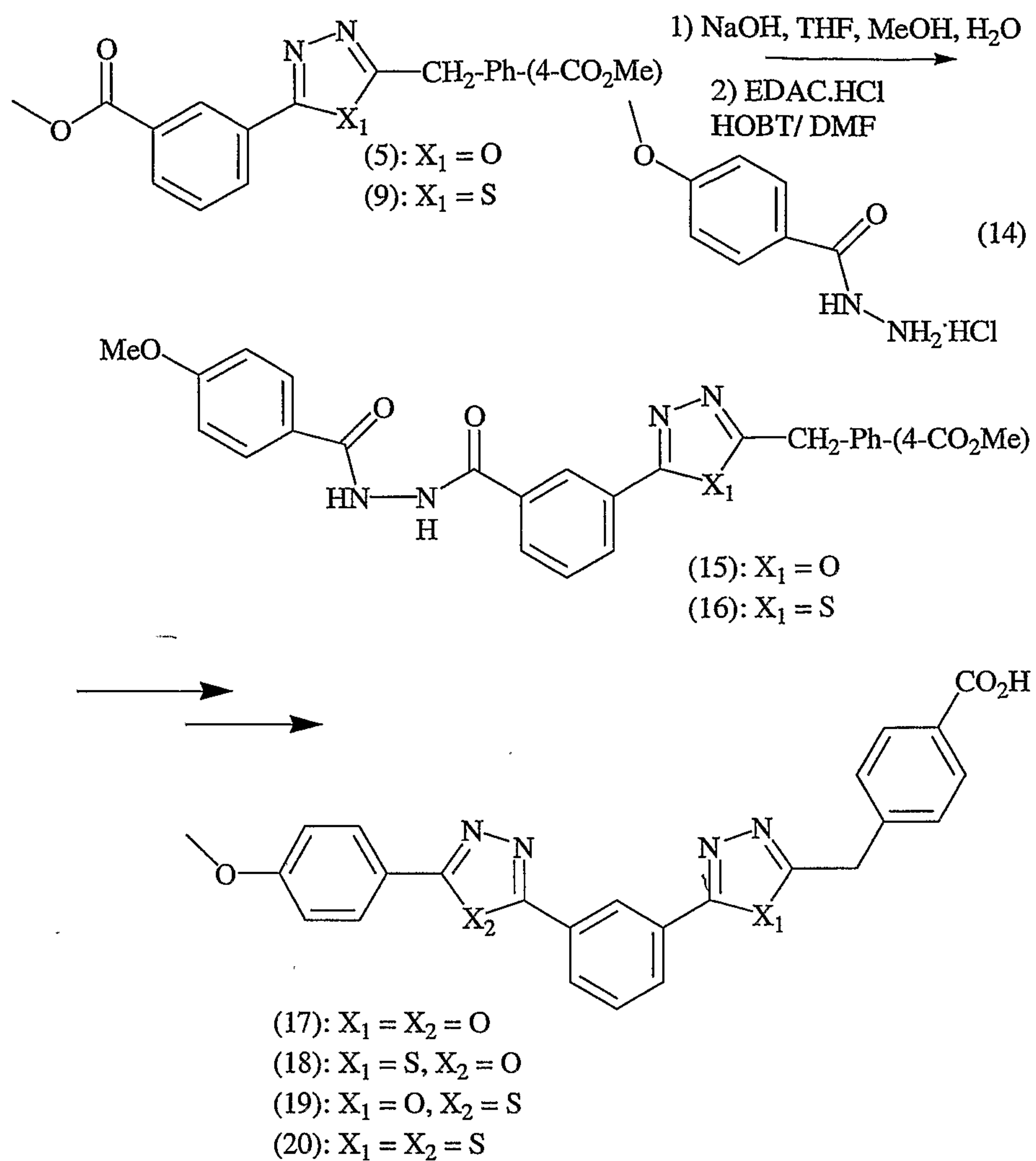
Scheme 9a.
