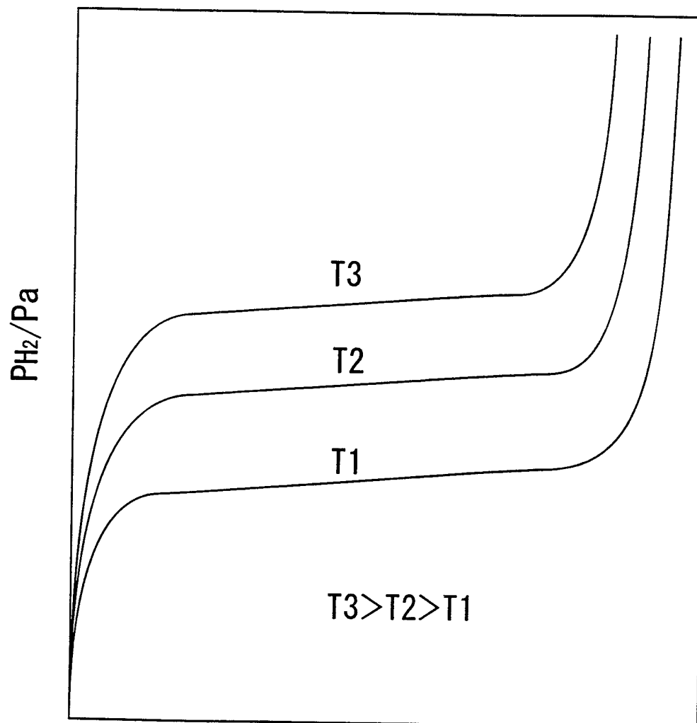
LaNi 5 系などにおける典型的な 水素解離曲線と温度の関係
