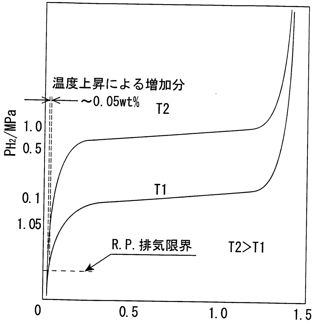
LaNi 5 系などにおける水素放出時の 温度上昇による放出量の変化
