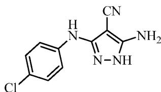
5-amino-3-((4-chlorophenyl)amino)-1 H -pyrazole-4-carbonitrile
