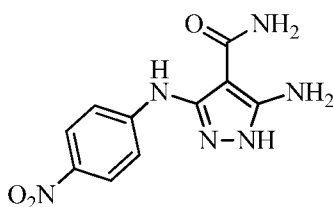
5-amino-3-((4-nitrophenyl)amino)-1 H -pyrazole-4-carboxamide
