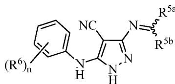
(XI-c)
