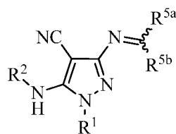
(VIII-b)
