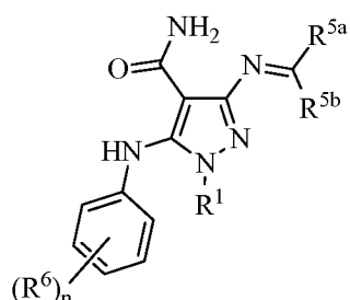
(XII-b)
