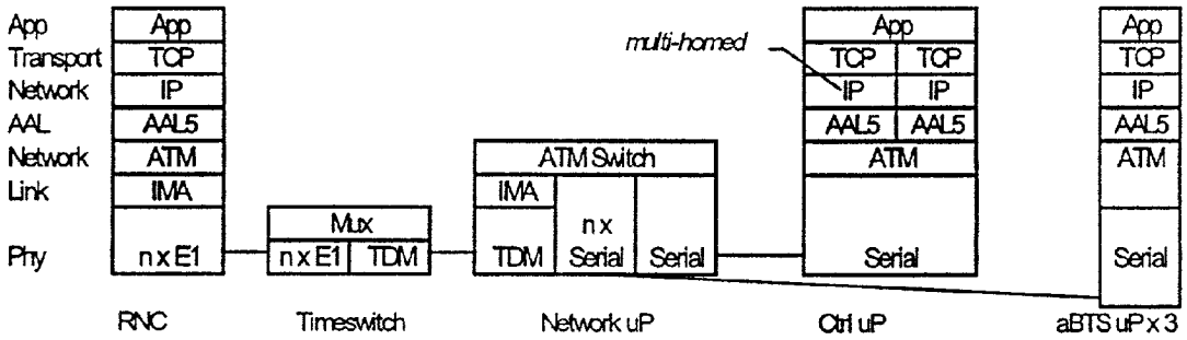
UMTS '99 (ATM backhaul) OMC-B Flow
