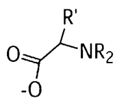
aminoacids
