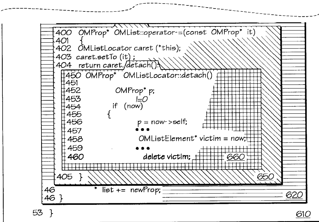
Fig. 6e
