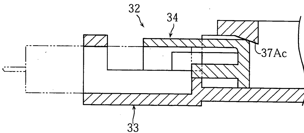
FIG.18B
