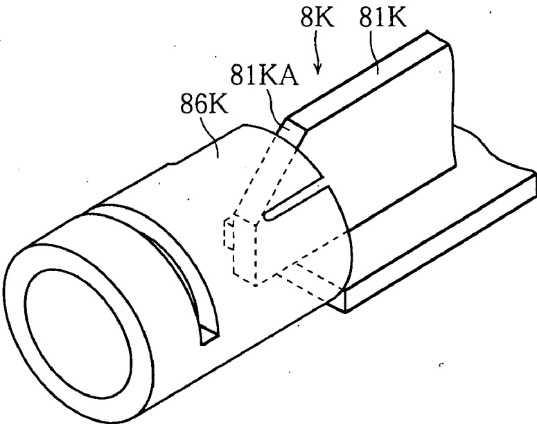
FIG.31A
