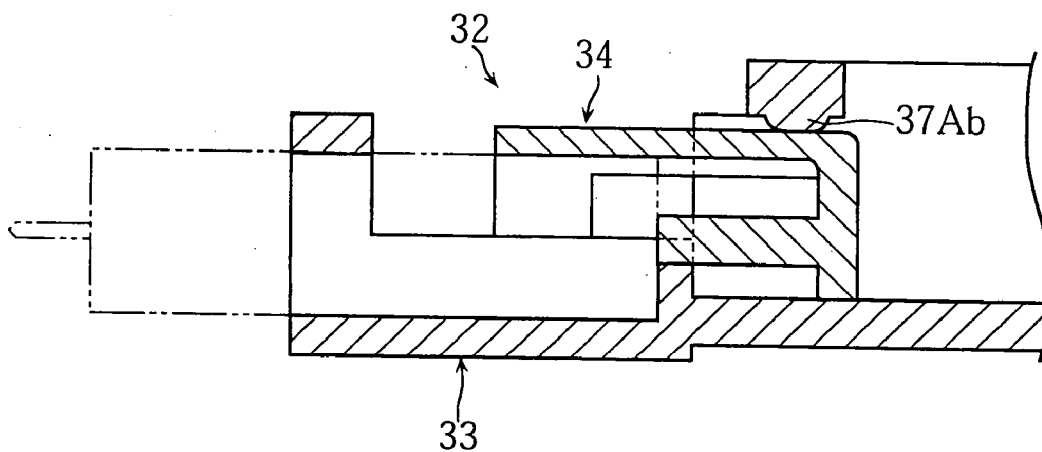
FIG.17C
