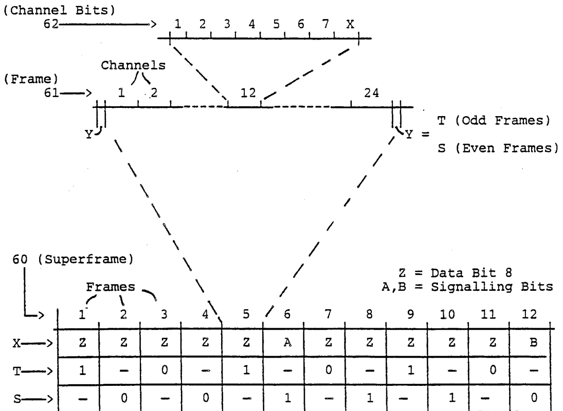
Fig. 7 (T-1 Frame Format)
