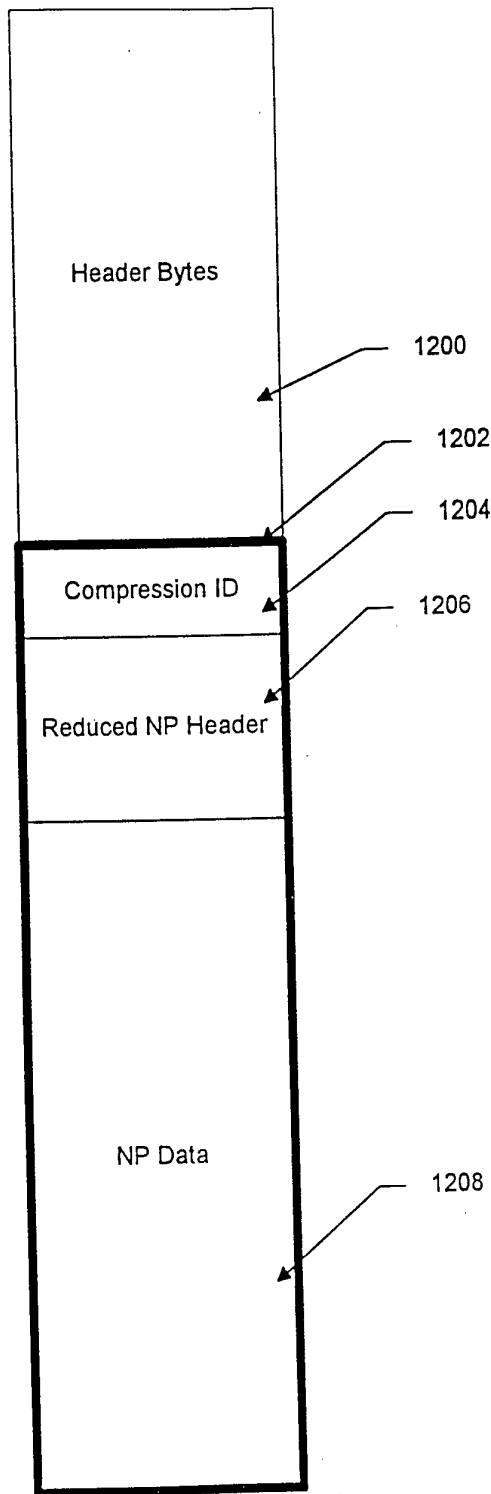
FIG. 12A
