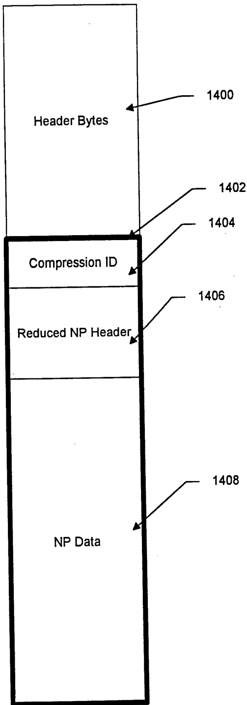
FIG. 14A
