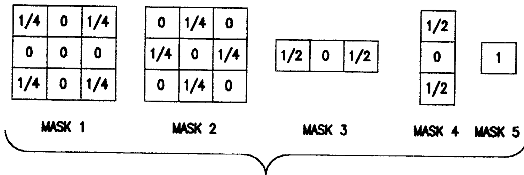
FIG. 12B
