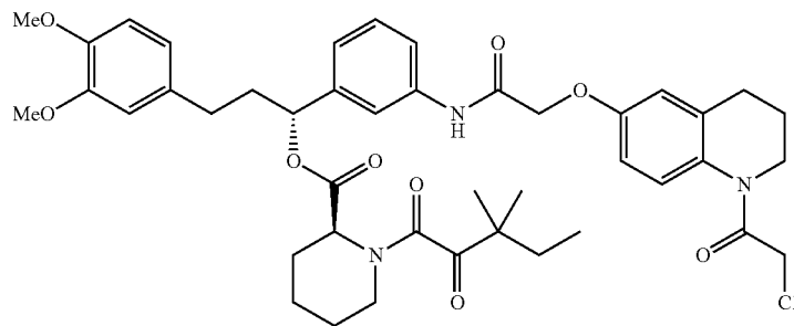
KB02-PEG0-SLF
