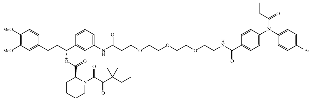
KB05-SLF
