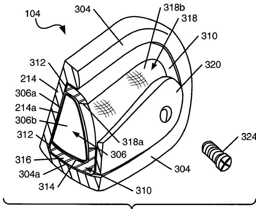
FIG. 3C
