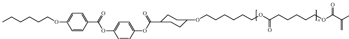
n \sim 9.6 1-(6-(6-(6-(6-(6-(6-(6-(6-(6-(trans-4-(4-hexyloxybenzoyloxy)phenoxy)carbonyl)cyclohexyloxy)hexyloxy)-6-oxohexyloxy)-6-oxohexyloxy)-6-oxohexyloxy)-6-oxohexyloxy)-6-oxohexyloxy)-6-oxohexyloxy)-6-oxohexyloxy)-2-methylprop-2-en-1-one
