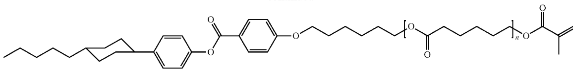
n \sim 6 1-(6-(6-(6-(6-(6-(6-(4-(4-(trans-4-pentylcyclohexyl)phenoxy)carbonyl)phenoxy)hexyloxy)-6-oxohexyloxy)-6-oxohexyloxy)-6-oxohexyloxy)-6-oxohexyloxy)-2-methylprop-2-en-1-one
