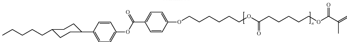
n \sim 1.8 1-(6-(6-(6-(4-(trans-4-pentylcyclohexyl)phenoxy)carbonyl)phenoxy)hexyloxy)-6-oxohexyloxy)-6-oxohexyloxy)-2-methylprop-2-en-1-one
