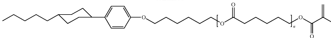
1-(6-(6-(6-(6-(4-(4-(trans-4-pentylcyclohexyl)phenoxy)hexyloxy)-6-oxohexyloxy)-6-oxohexyloxy)-6-oxohexyloxy)-2-methylprop-2-en-1-one
