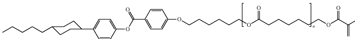
n \sim 7.5 1-(6-(6-(6-(6-(6-(6-(6-(4-(4-(trans-4-pentylcyclohexyl)phenoxycarbonyl)phenoxy)hexyloxy)-6-oxohexyloxy)-6-oxohexyloxy)-6-oxohexyloxy)-6-oxohexyloxy)-6-oxohexyloxy)-6-oxohexyloxy)-2-methylprop-2-en-1-one
