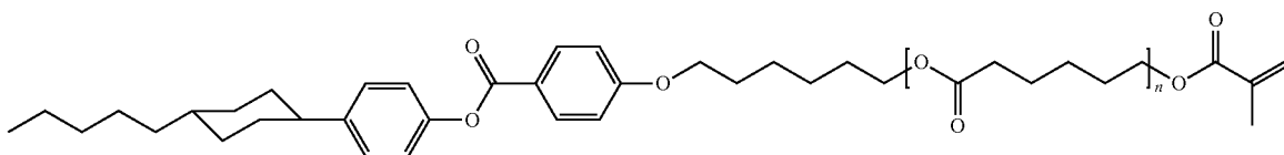
n \sim 2.1 1-(6-(6-(6-(4-trans-4-pentylcyclohexyl)phenoxy)carbonyl)phenoxy)hexyloxy)-6-oxohexyloxy)-2-methylprop-2-en-1-one
