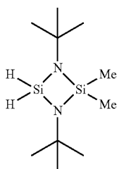
1,3-bis(tert-butyl)-2- dimethylcyclodisilazane
