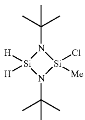
1,3-bis(tert-butyl)-2-chloro-2- methylcyclodisilazane
