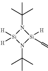
1,3-bis(tert-butyl)-2-ethynyl cyclodisilazane
