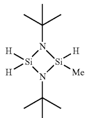
1,3-bis(tert-butyl)-2-methylcyclodisilazane
