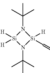
1,3-bis(tert-butyl)-2-vinylcyclodisilazane
