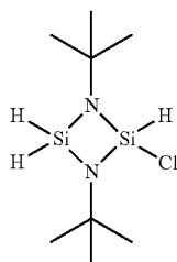
1,3-bis(tert-butyl)-2-chlorocyclodisilazane
