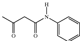
Acetoacetanilide
