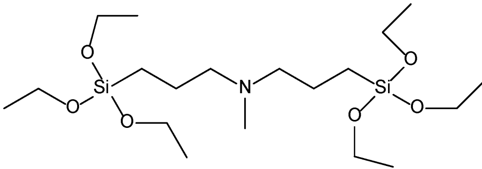
- 2-[Bis[3-(triethoxysilyl)propyl]amino]-ethanol
