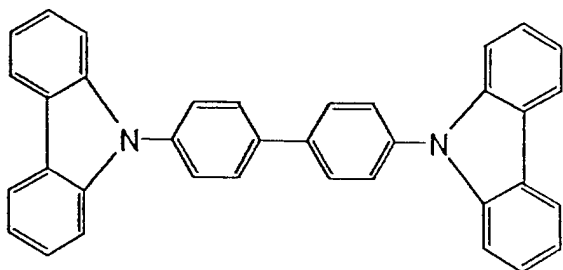
CBP
