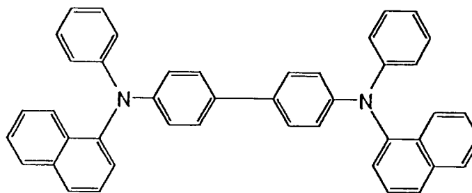
\alpha -NPD
