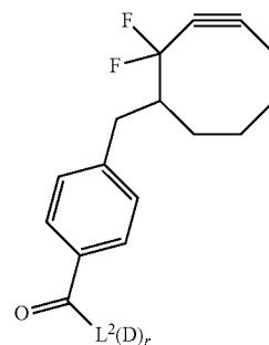
DIFO2- L^2(D)_r
