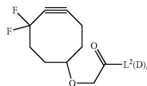
DIFO- L^2(D)_r
