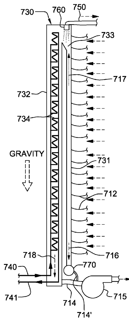
FIG. 7C
