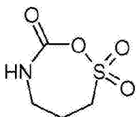
化合物 D1
