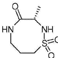
化合物 D7
