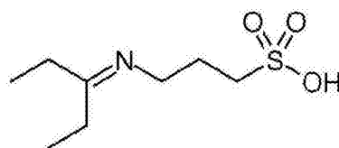
化合物 M2
