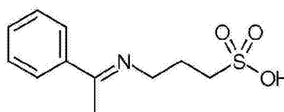
化合物 M6
