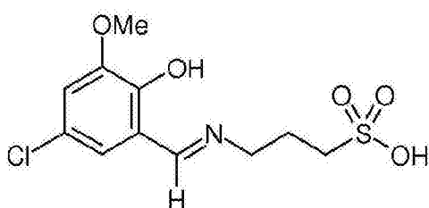
化合物 M9
