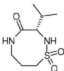
化合物 D8
