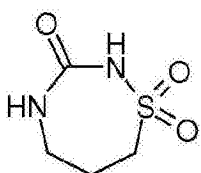
化合物 D5
