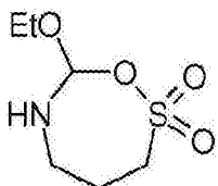
化合物 D3
