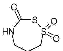
化合物 D6
