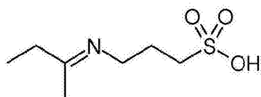
化合物 M3
