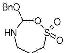
化合物 D4
