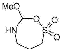
化合物 D2
