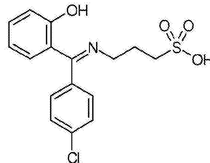
化合物 M8
