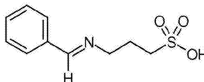
化合物 M4
