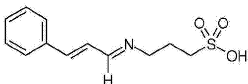
化合物 M5
