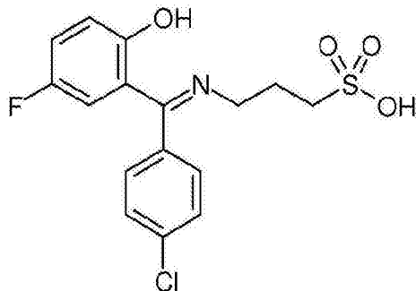
化合物 M7
