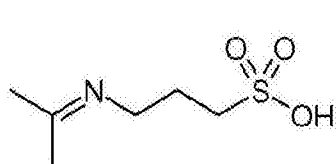
化合物 M1
