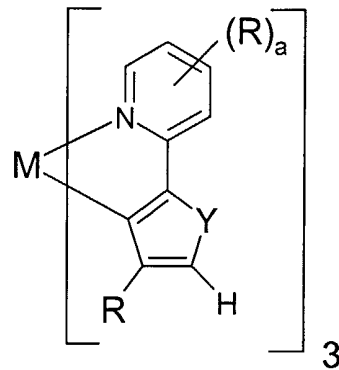
Verbindungen (IV)
