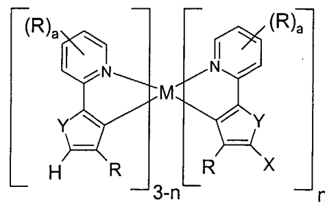
Verbindungen (II)
