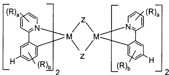
Verbindungen (VI)
