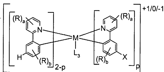
Verbindungen (XIII)
