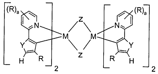
Verbindungen (VIII)
