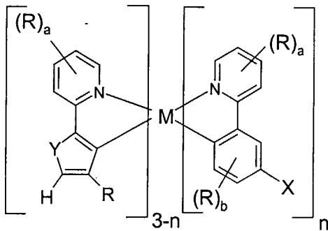
Verbindungen (Ia)
