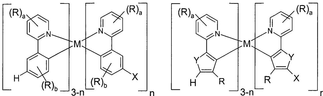
Verbindungen (I)
