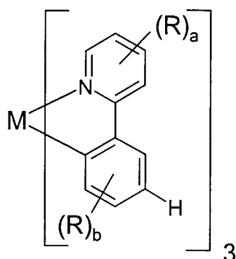
Verbindungen (III)
