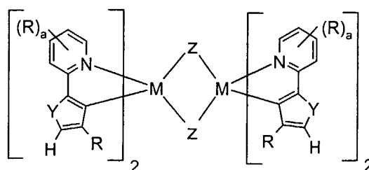
Verbindungen (VIII)
