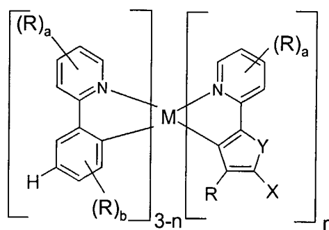
Verbindungen (IIa)
