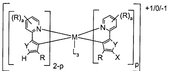
Verbindungen (XV)
