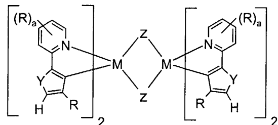
Verbindungen (VIII)
