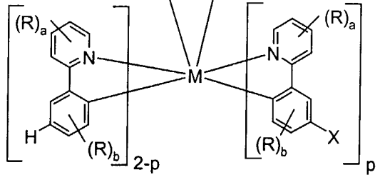
Verbindungen (V)
