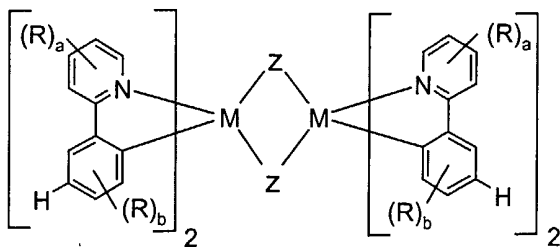
Verbindungen (VI)
