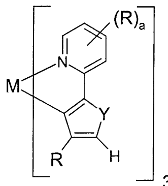
Verbindungen (IV)
