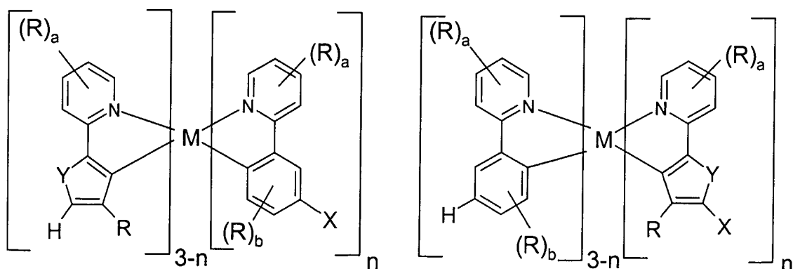
Verbindungen (Ia)
