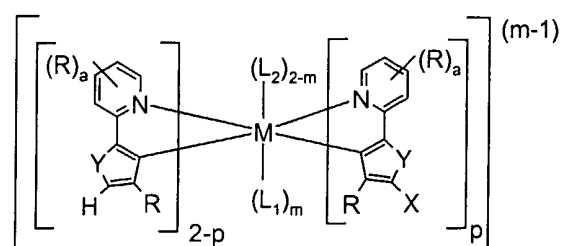
Verbindungen (XI)
