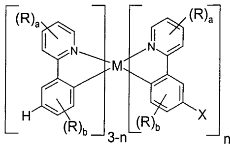
Verbindungen (I)
