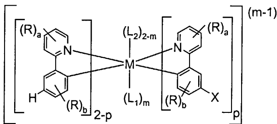
Verbindungen (IX)
