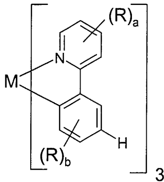
Verbindungen (III)
