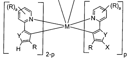
Verbindungen (VII)
