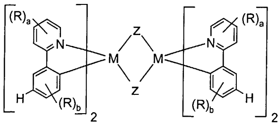
Verbindungen (VI)
