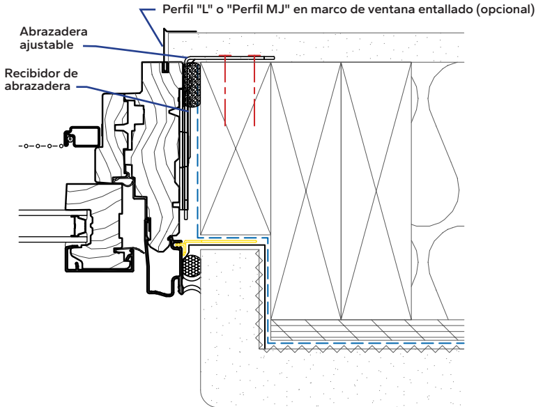
Enmarcado empotrado de 2 x 4 dentro de una estructura de pared de 2 x 6
